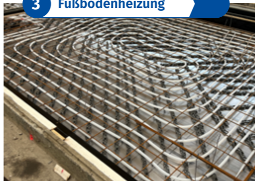
3 Fußbodenheizung
